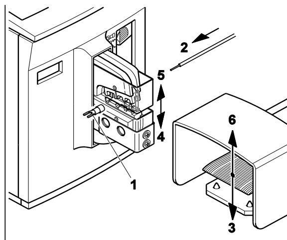
Рисунок 11 Опрессовка кабельных наконечников
