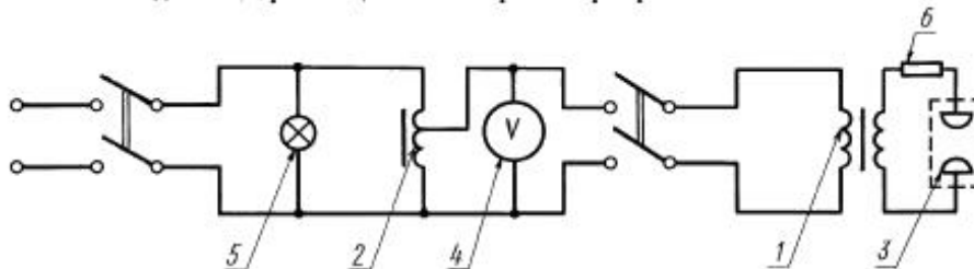
Принципиальная схема установки для определения пробивного напряжения жидких электроизоляционных материалов при промышленной частоте
